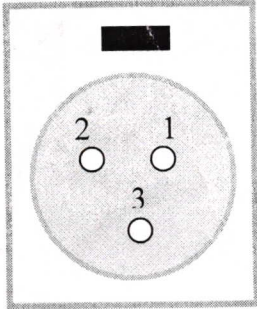
Steckdose 24V Frontansicht
