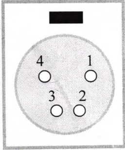
Steckdose 12V Frontansicht
